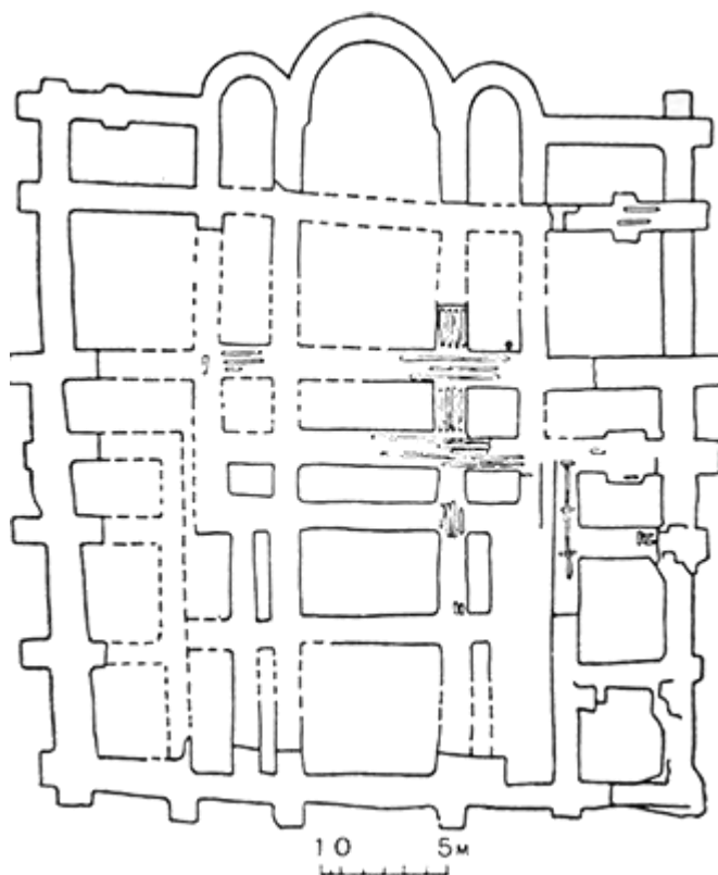
План фундаментів Десятинної церкви.
