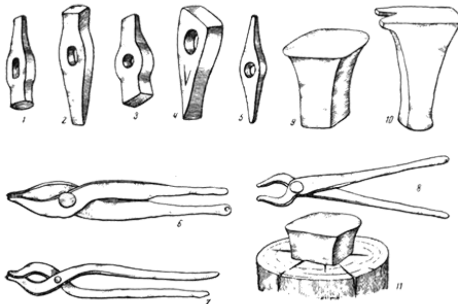
Ковальські інструменти. 1,2 – молотки-ручніки; 3,4 – молотки-сікачі; 5 – молоток для тонкої роботи; 6–8 – кліщі; 9 – ковадло просте; 10 – ковадло з розтрубом; 11 – ковадло на колоді.
