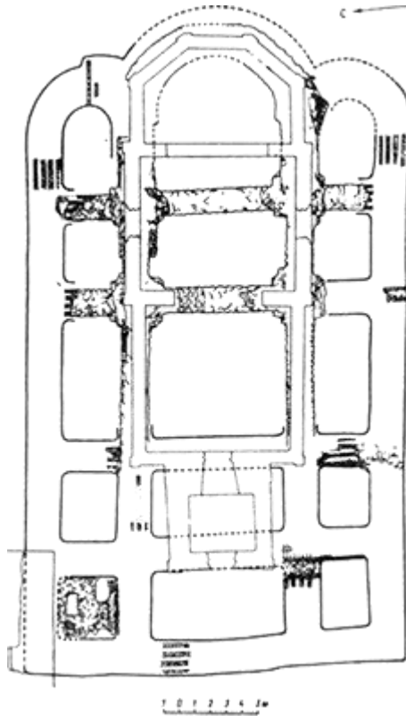
План фундаменту церкви Бориса і Гліба у Вишгороді.
