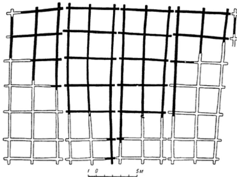
План внутрівальних клітей города Ярослава.
